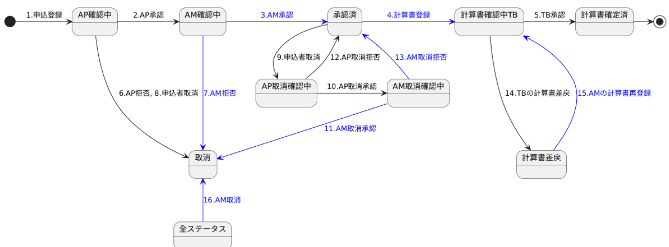
Figure 1. ステータス遷移図: AMが操作可能な部分は青色で表示。
